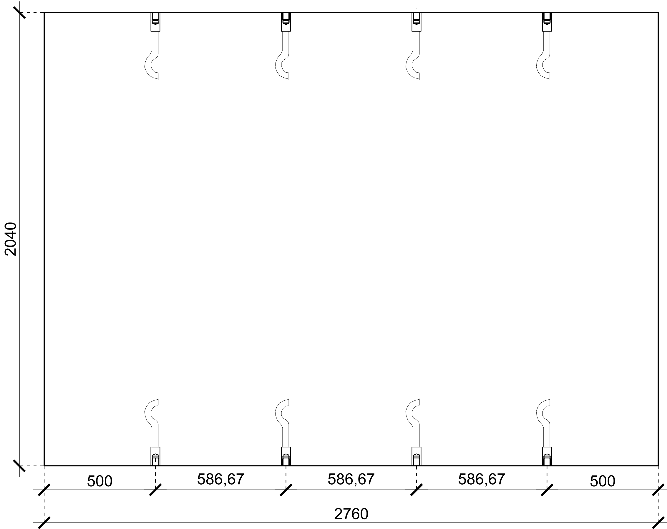
Feneklemez Lemezvastagság: 150 mm Készül: 1 db
