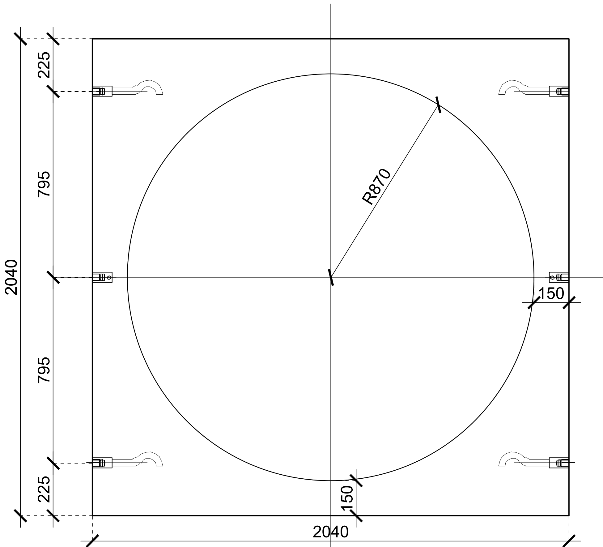
Csövet fogadó lemez Lemezvastagság: 150 mm Készül: 1 db
