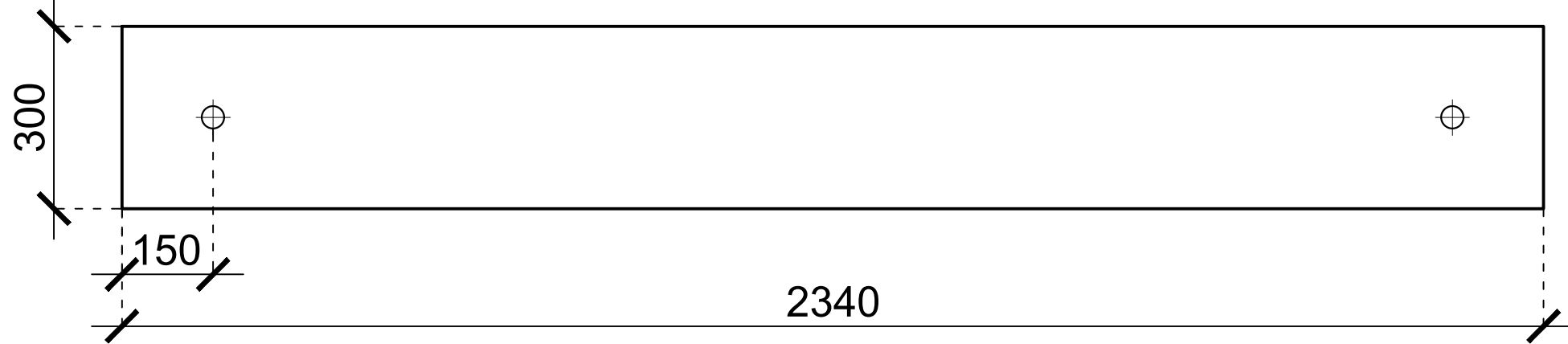
Felső összefogó lemez Lemezvastagság: 150 mm Készül: 1 db
