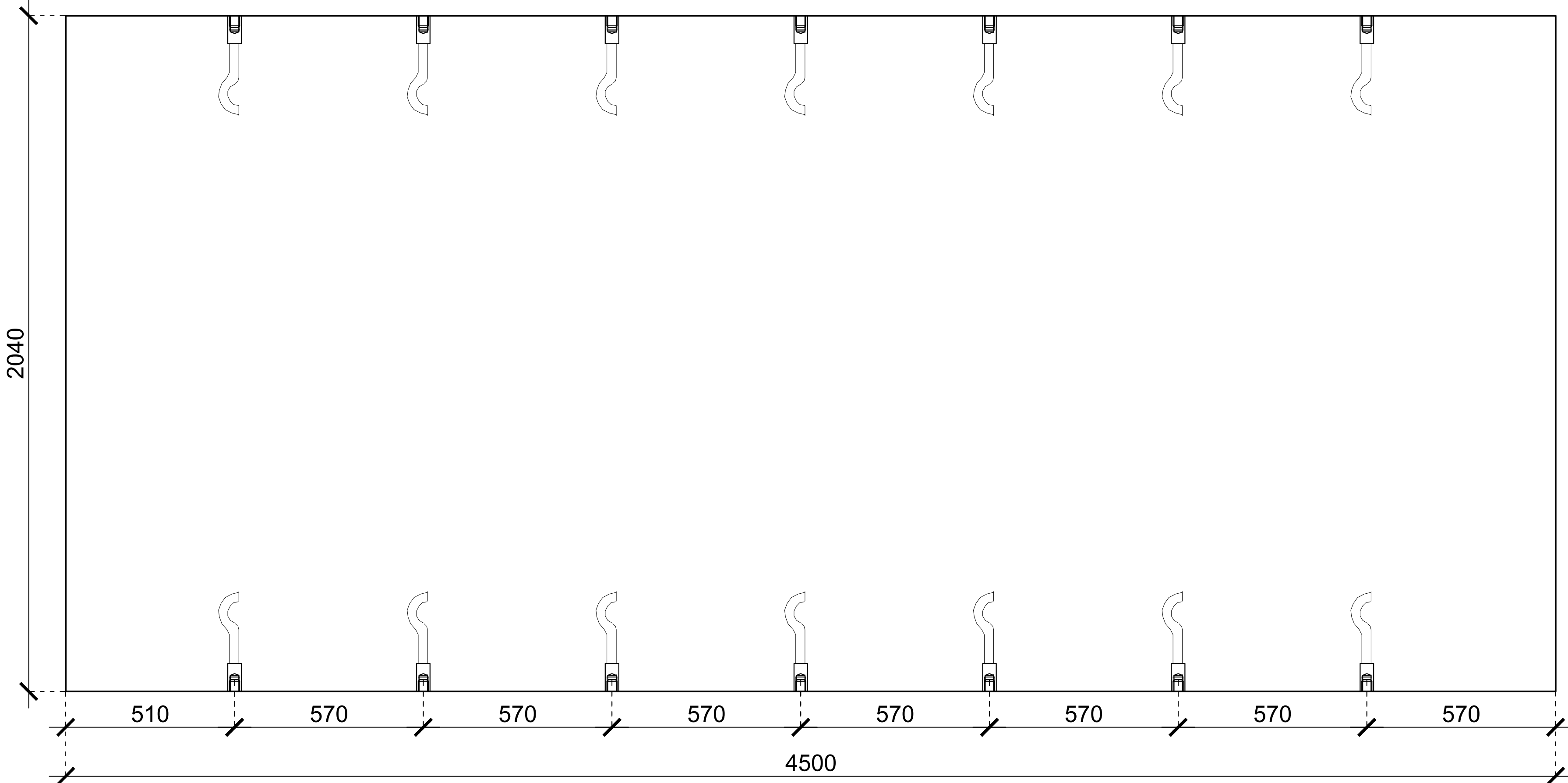
Feneklemez Lemezvastagság: 150 mm Készül: 1 db
