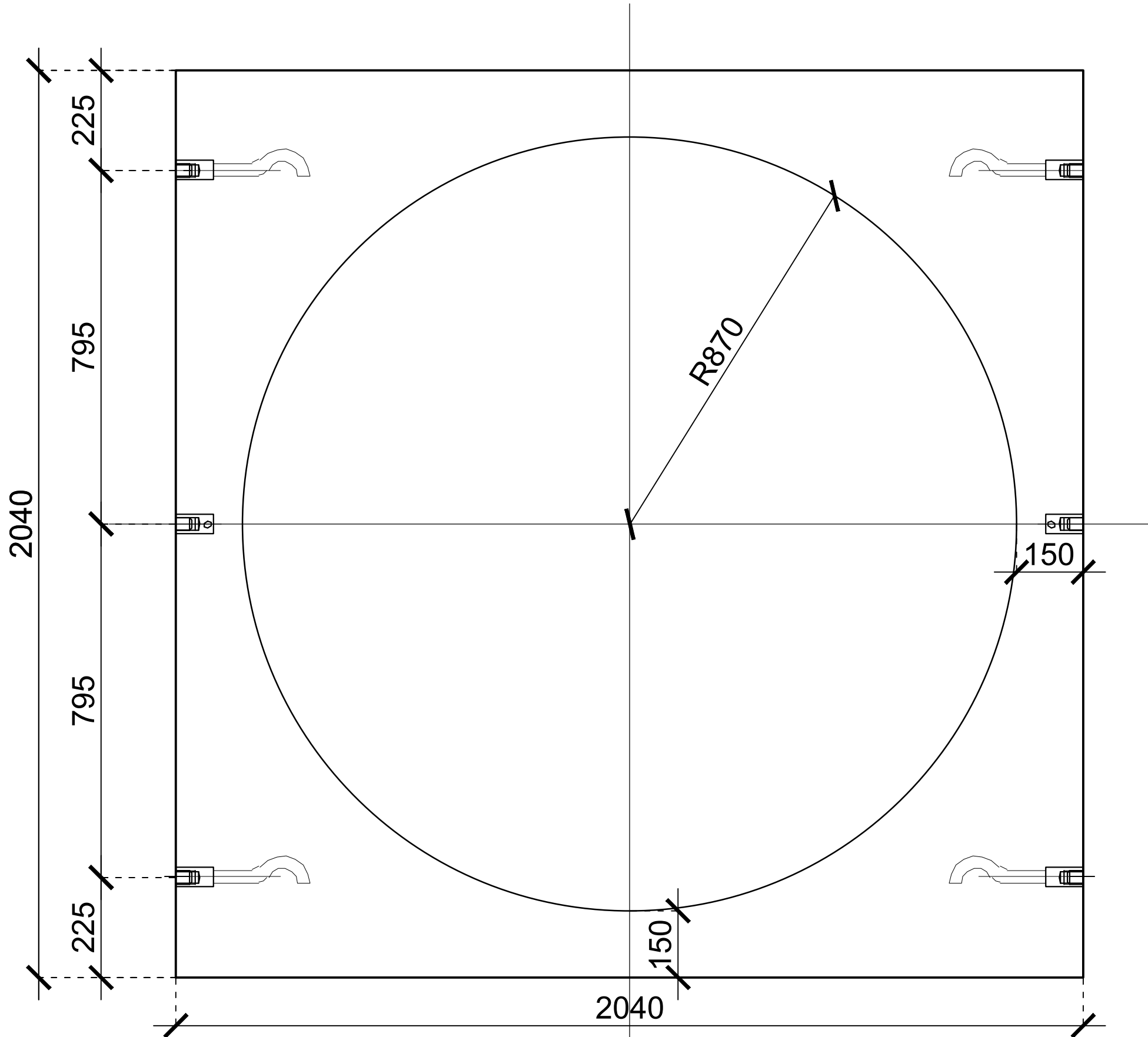
Csővet fogadó lemez Lemezvastagság: 150 mm Készül: 1 db
