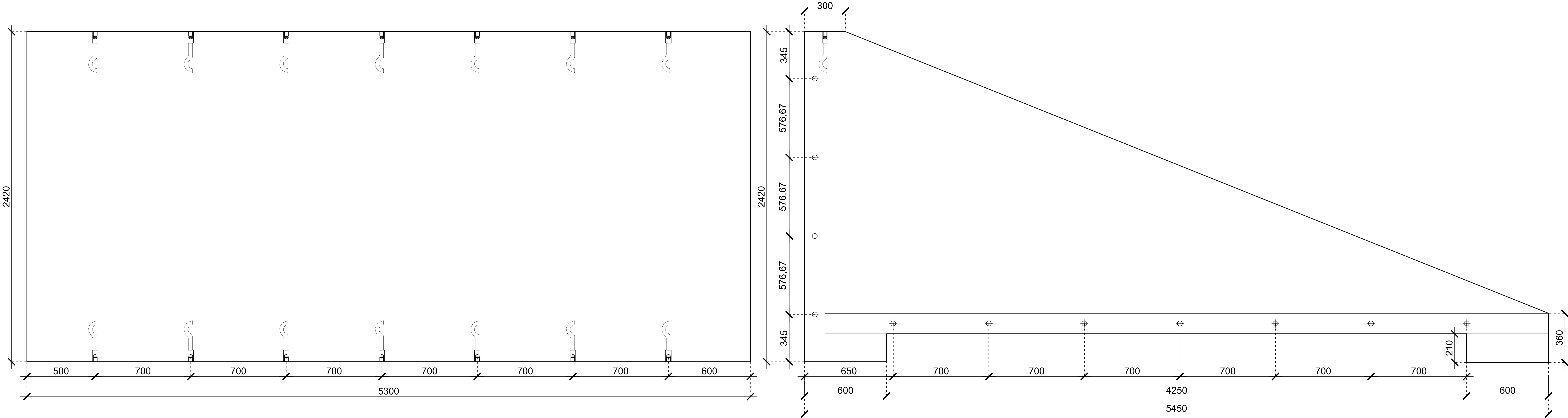
Oldallemez Lemezvastagság: 150 mm Készül: 2 db
