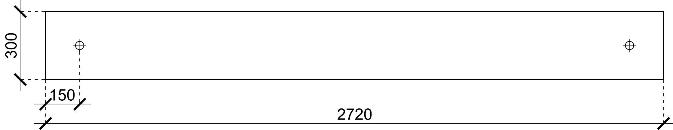
Felső összefogó lemez Lemezvastagság: 150 mm Készül: 1 db
