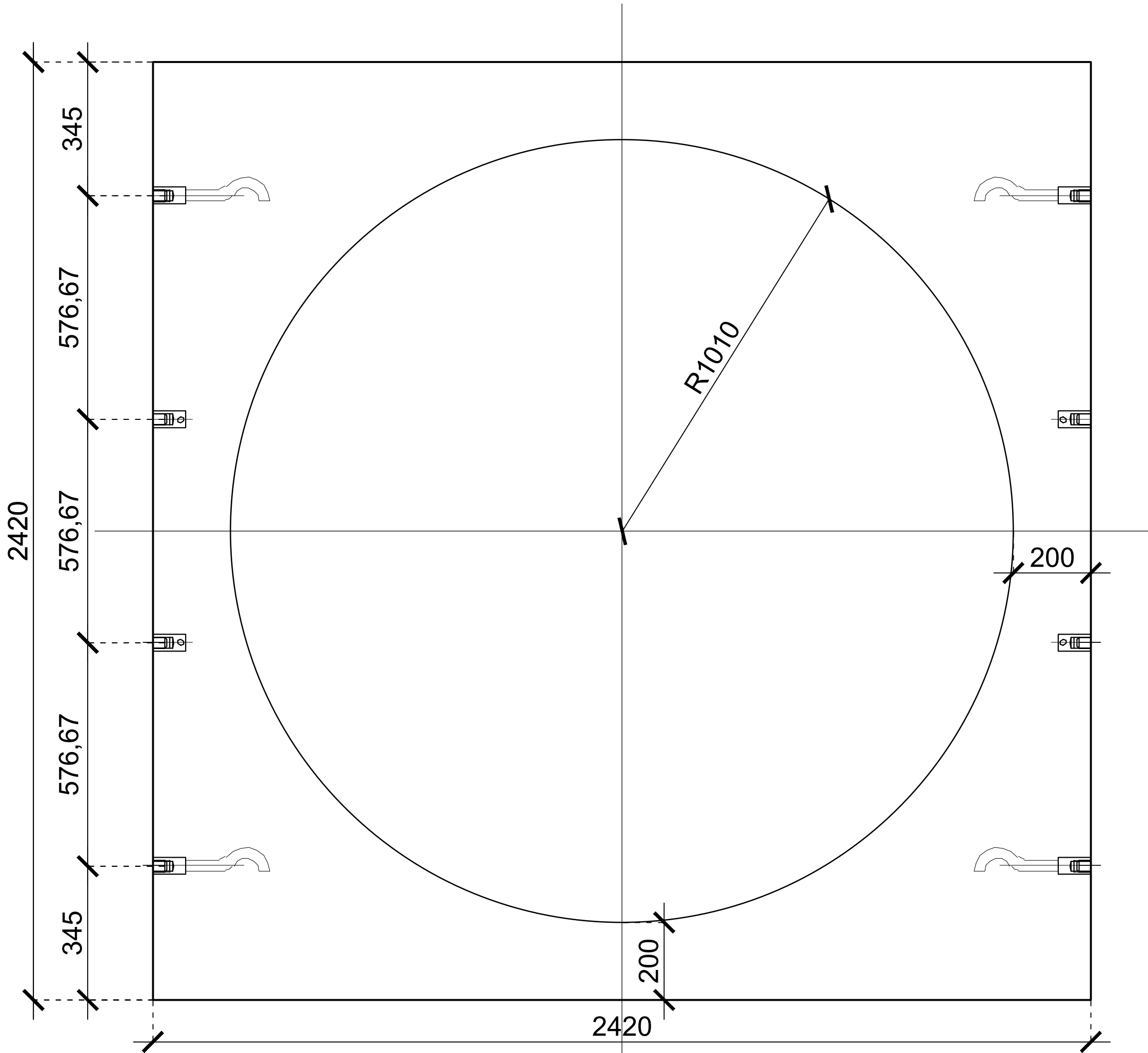
Csővet fogadó lemez Lemezvastagság: 150 mm Készül: 1 db
