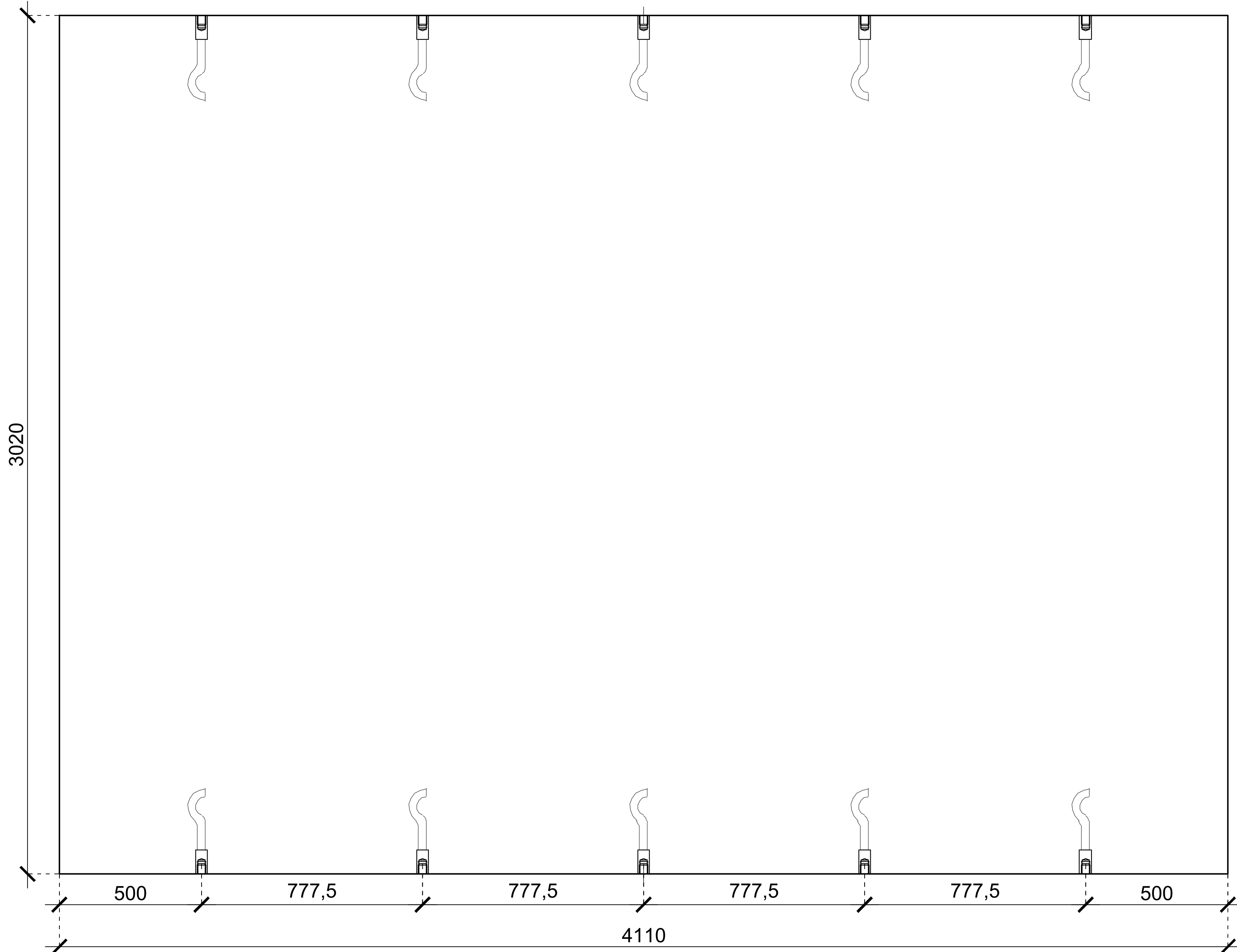
Fenéklemez Lemezvastagság: 150 mm Készül: 1 db
