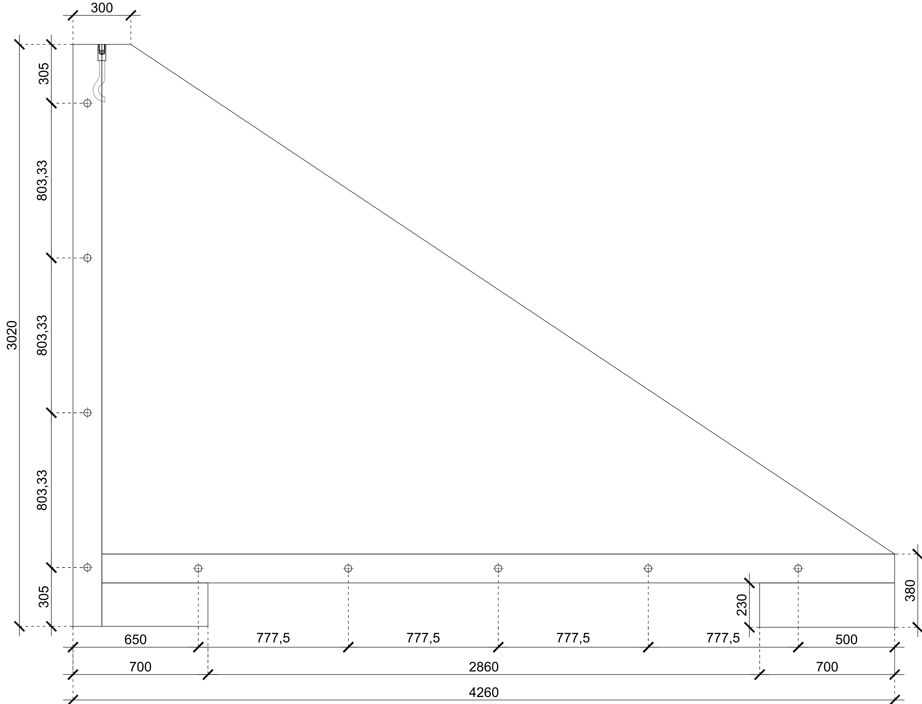
Oldallemez Lemezvastagság: 150 mm Készül: 2 db
